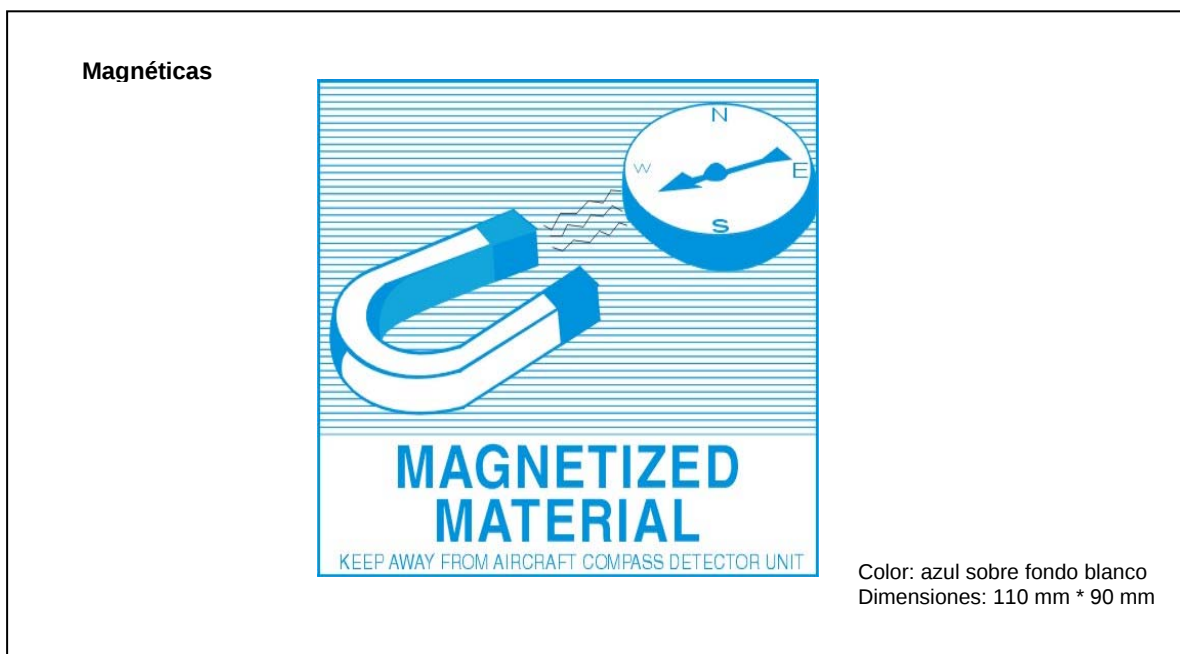
Figura 5-22. Material magnetizado
