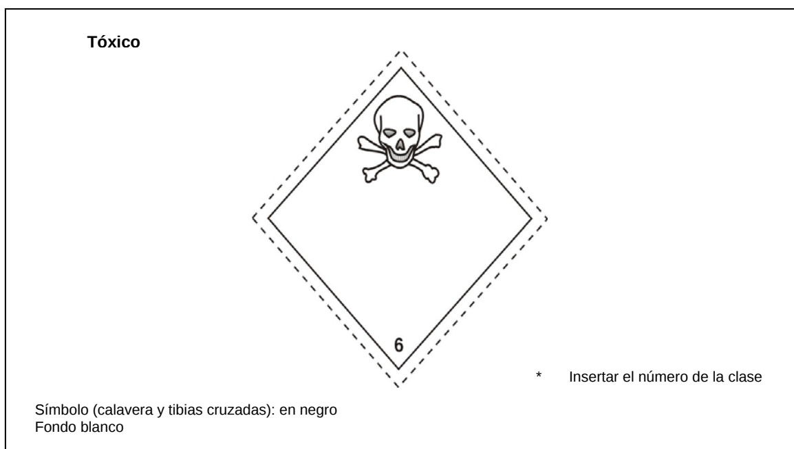
Figura 5-14. Sustancia tóxica; Clase 6, División 6.1
